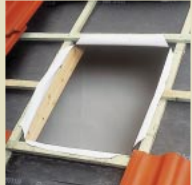
↑ Nun wird die Unterspann- oder Unterdeckeckbahn eingeschnitten und auf die Dachlattung umgelegt und befestigt.
